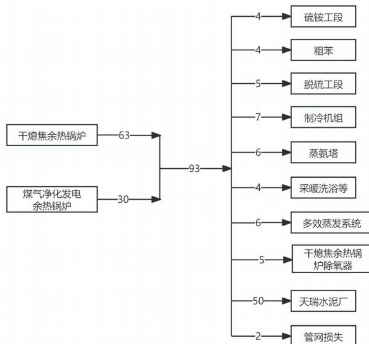
图 2-5 项目建成后全厂蒸汽平衡图 单位：t/h
