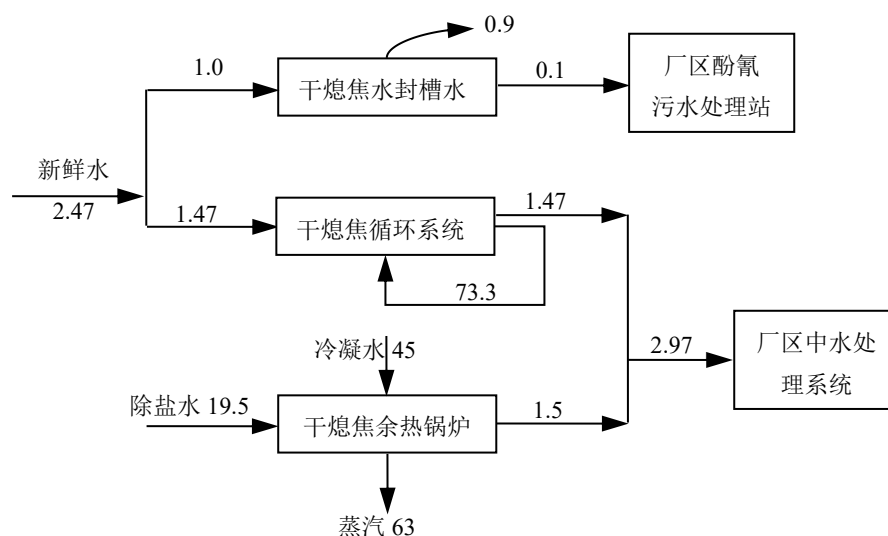
图 2-1 本项目水平衡示意图 单位： \text{m}^3/\text{h}
