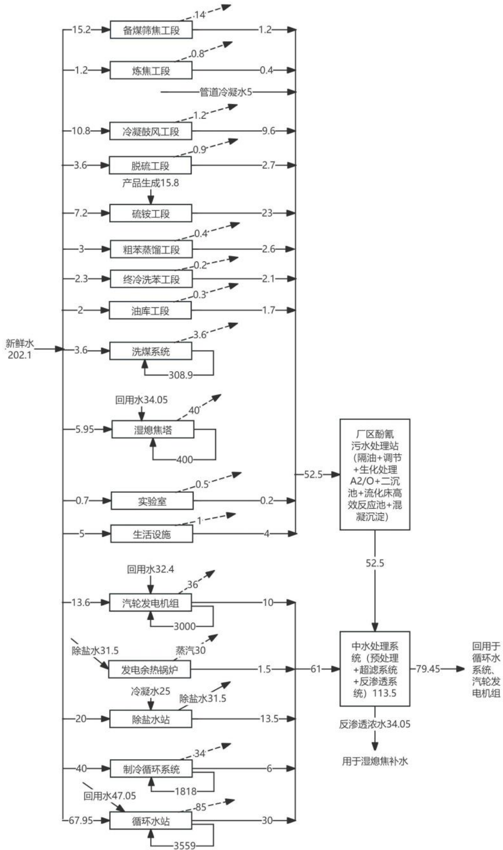
图 2-2 现有工程水平衡示意图 单位: m³/h
