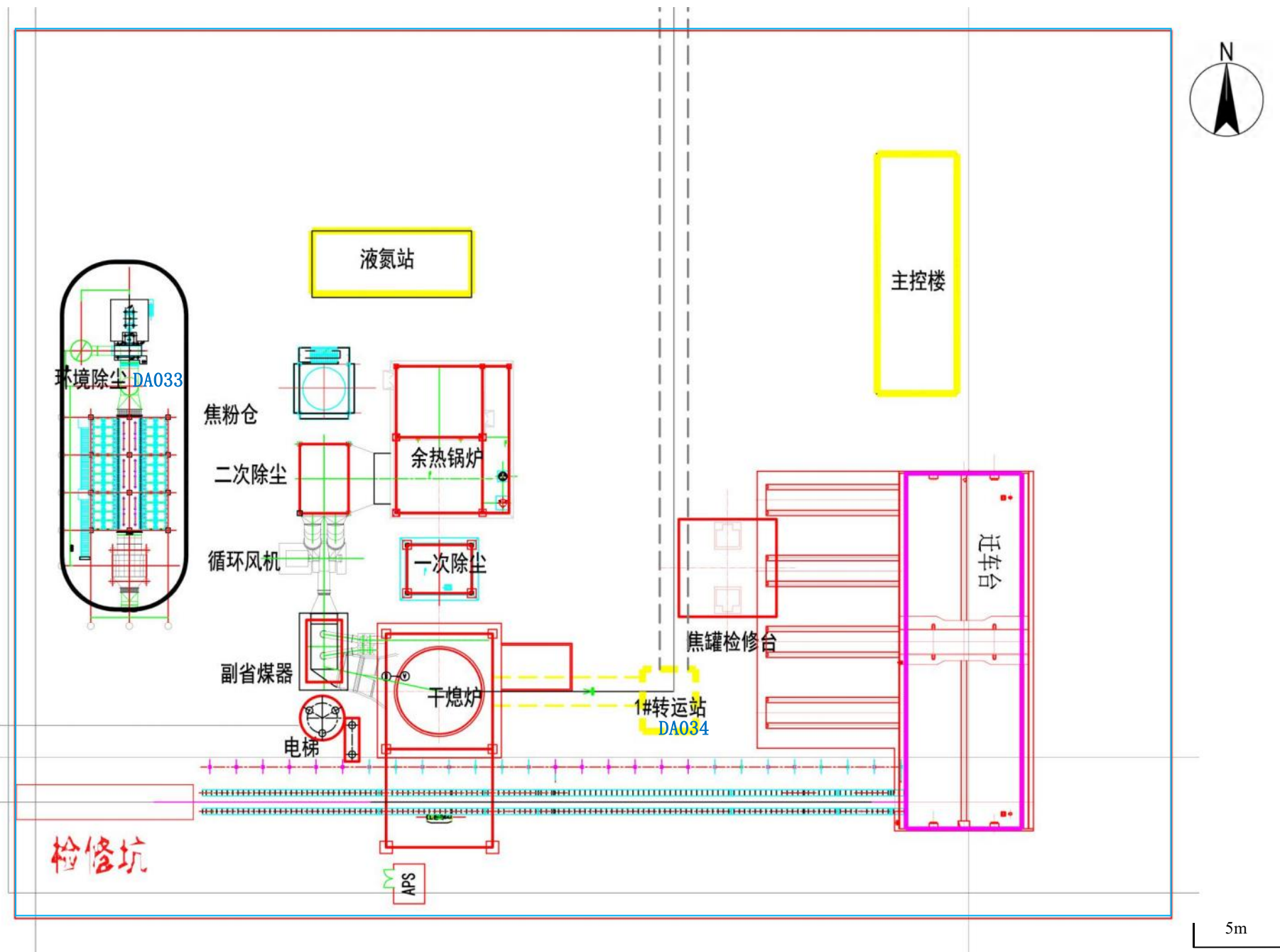
附图六 本项目平面布置图
