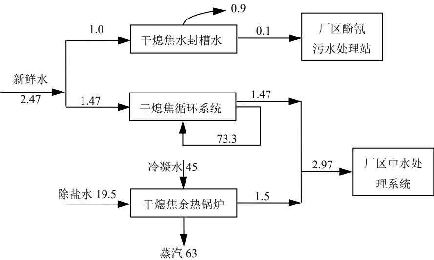
图 2-1 本项目水平衡示意图 单位：m³/h
