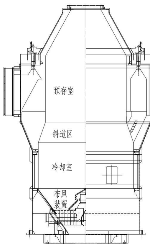
图 2-6 干熄炉示意图
