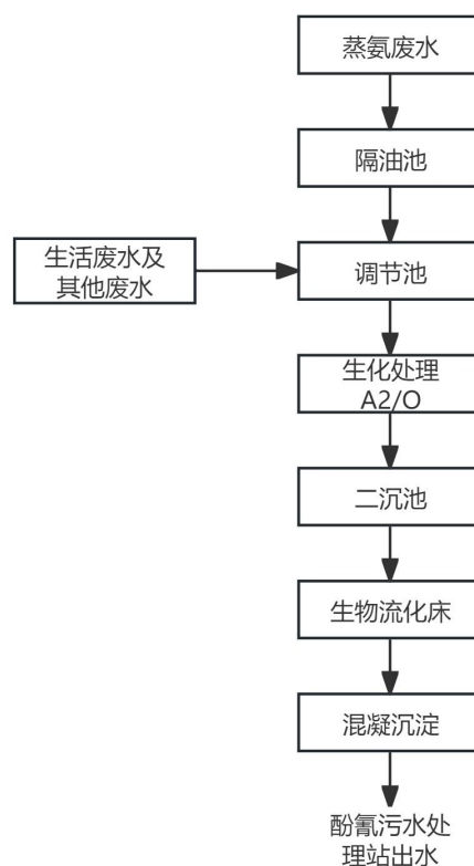
图 4-1 厂区酚氰污水处理站处理工艺示意图
