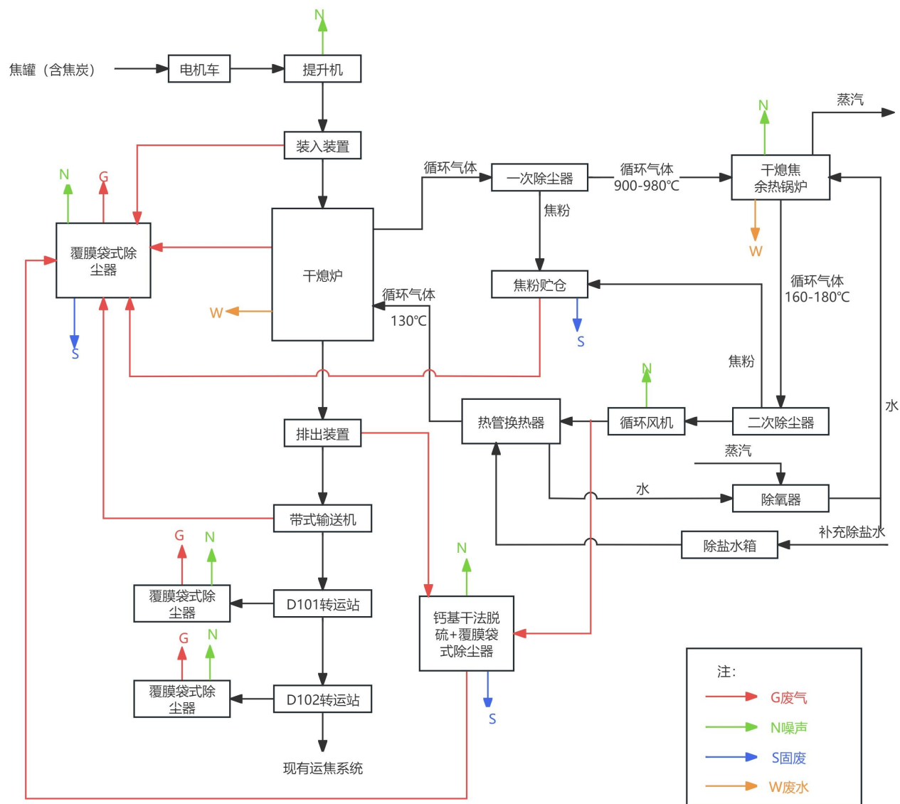
图 2-7 运营期干熄焦及余热利用工艺流程及产污节点图
