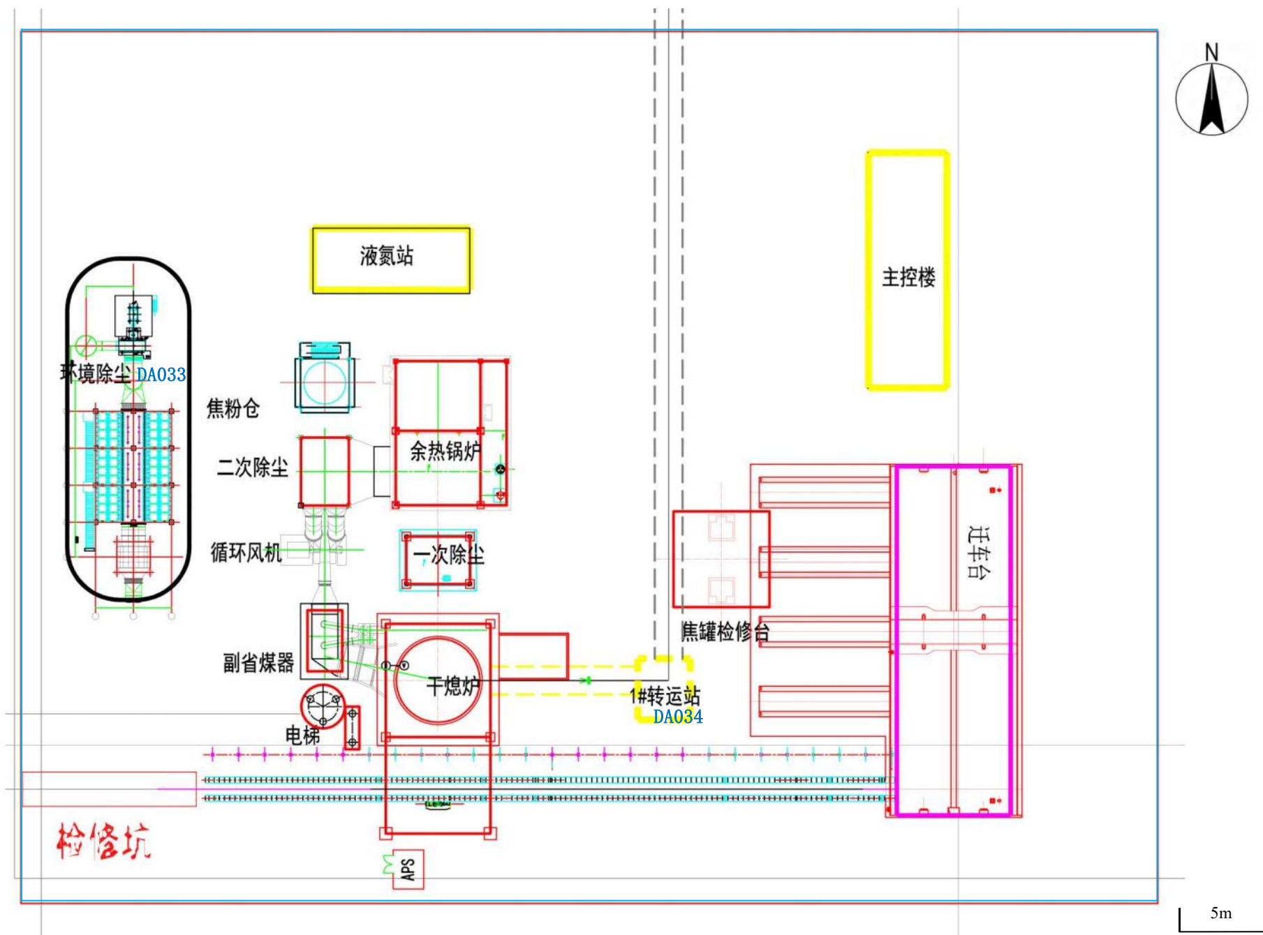
附图六 本项目平面布置图
