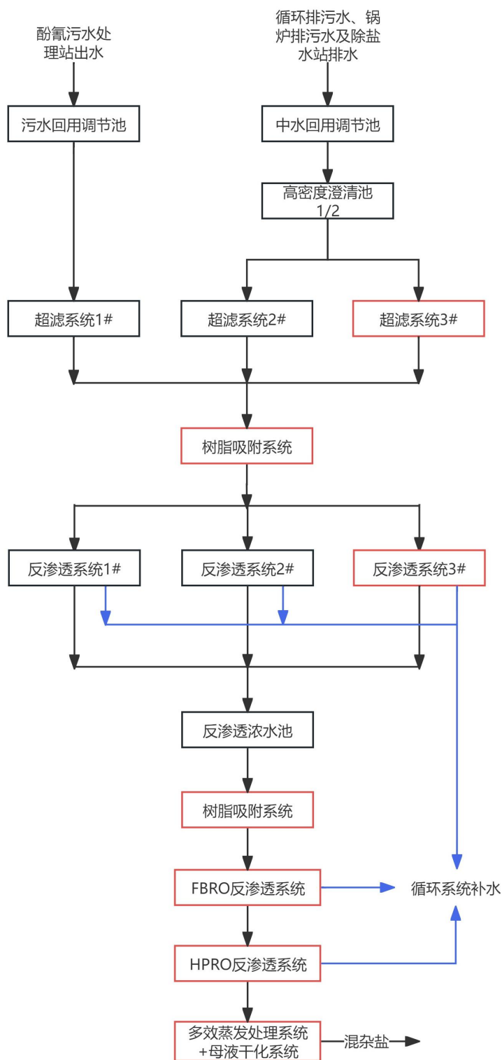
图 4-2 厂区中水处理系统及反渗透浓水处理工艺示意图（红框设施为新增）
