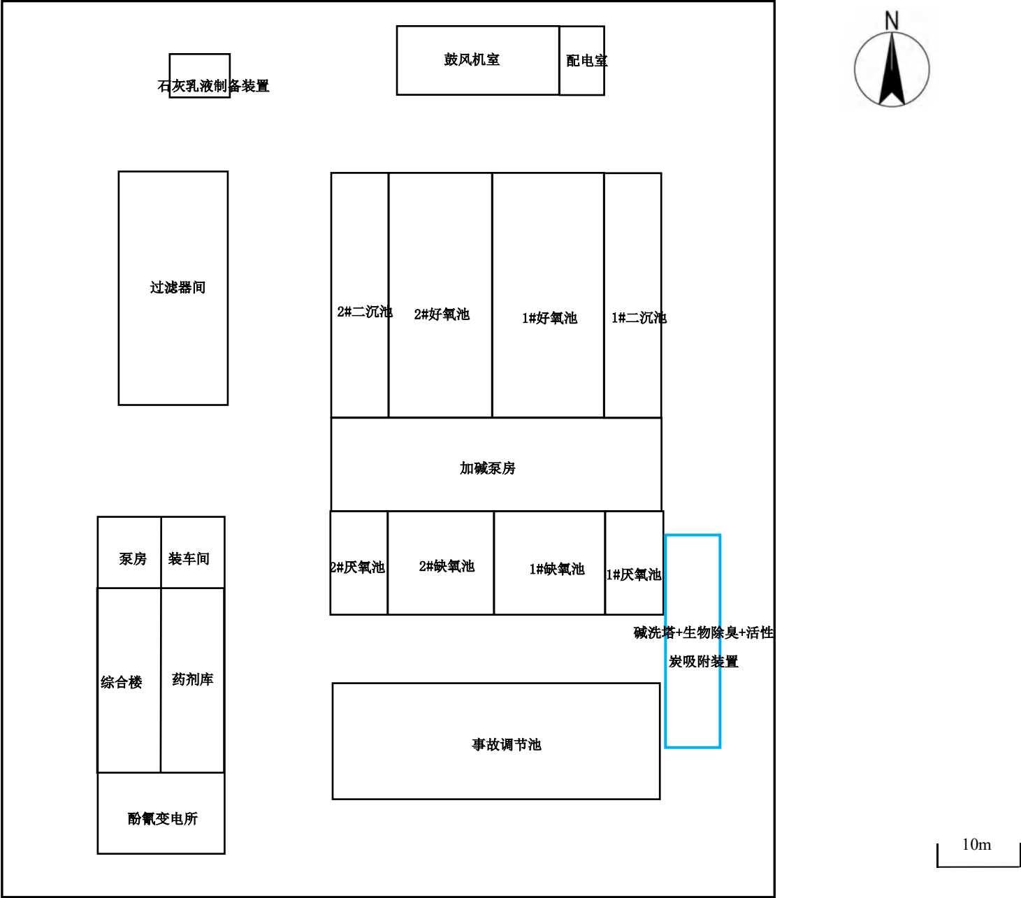
附图七 项目厂区污水处理站平面布置图（1）
