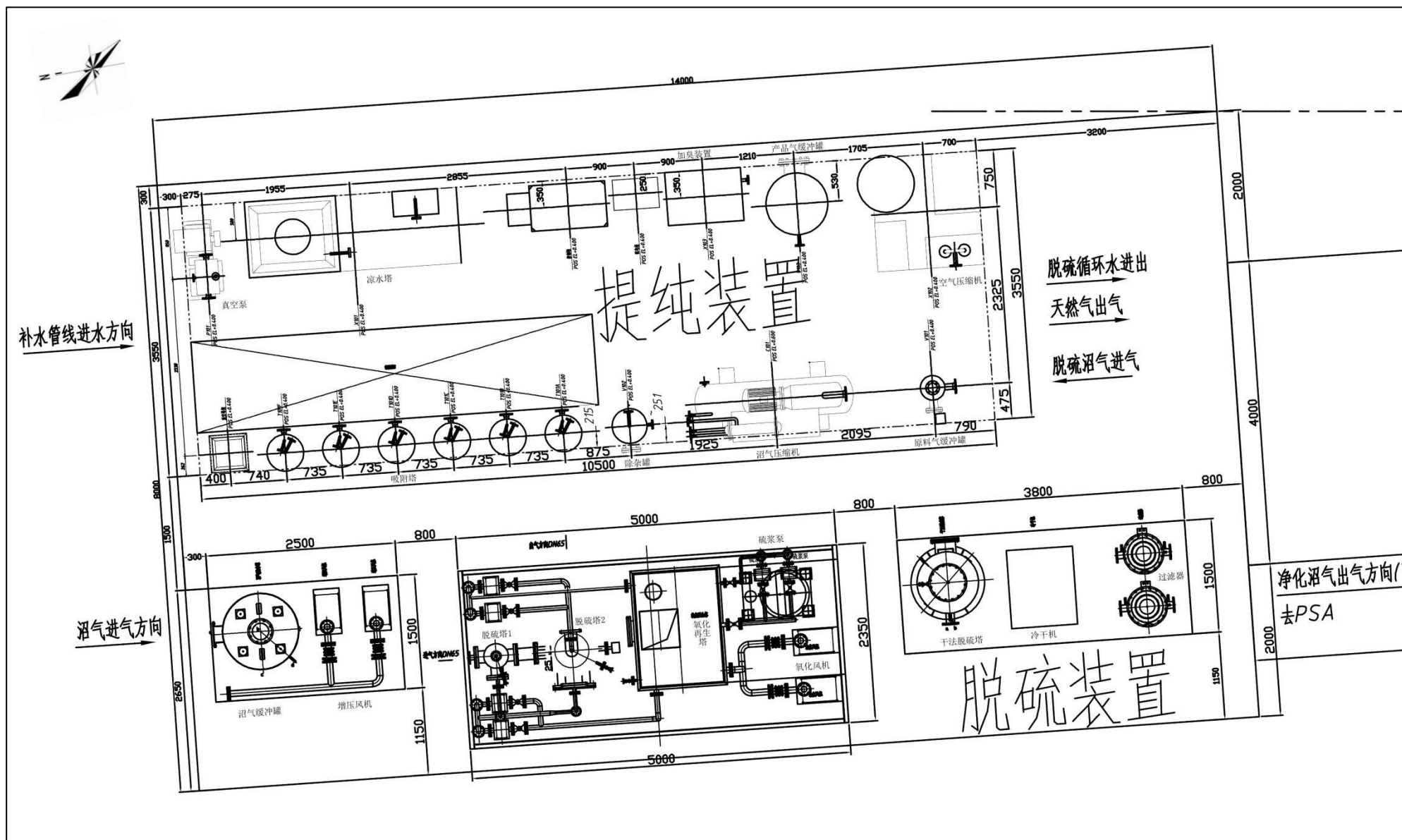
附图5 本项目设备布局图
