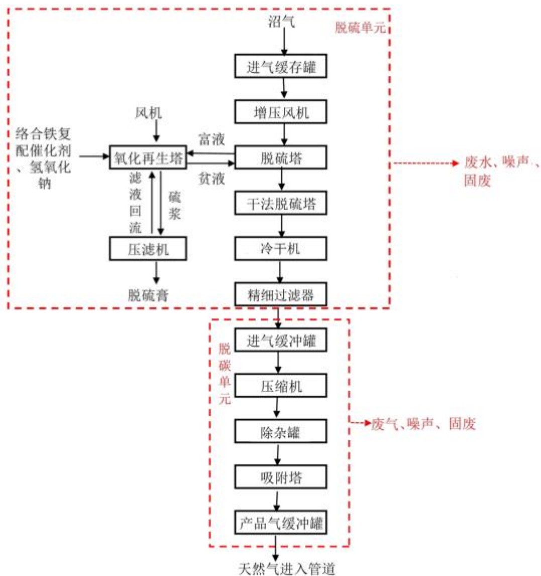
图 2-4 本项目工艺流程及产污环节示意图
